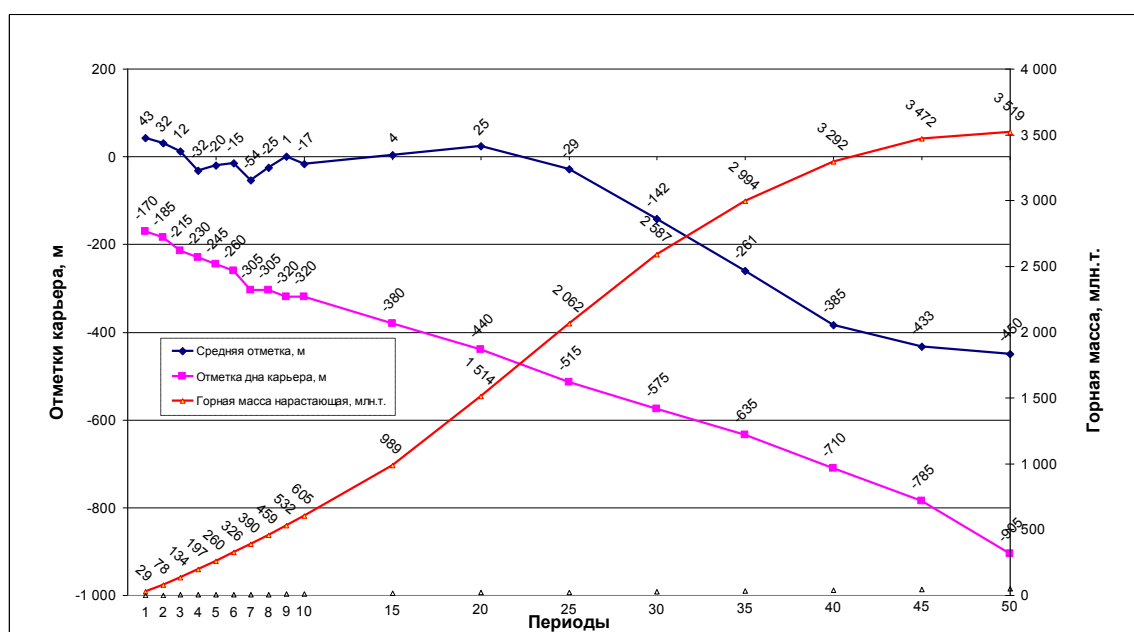
Рис. 2 – Графики изменения нарастающих объемов горной массы, отметки дна и средней отметки подъема горной массы по мере отработки оптимального карьера
