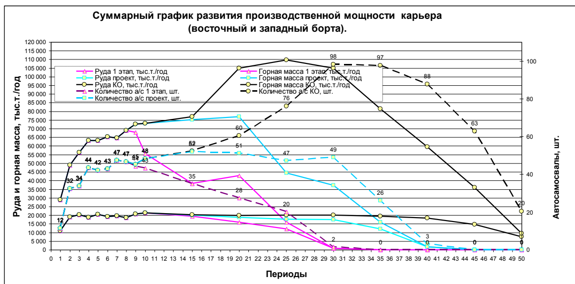
Рис. 1 – Графики развития производственной мощности в вариантах отработки этапа 1, проектного и оптимального контуров карьера
